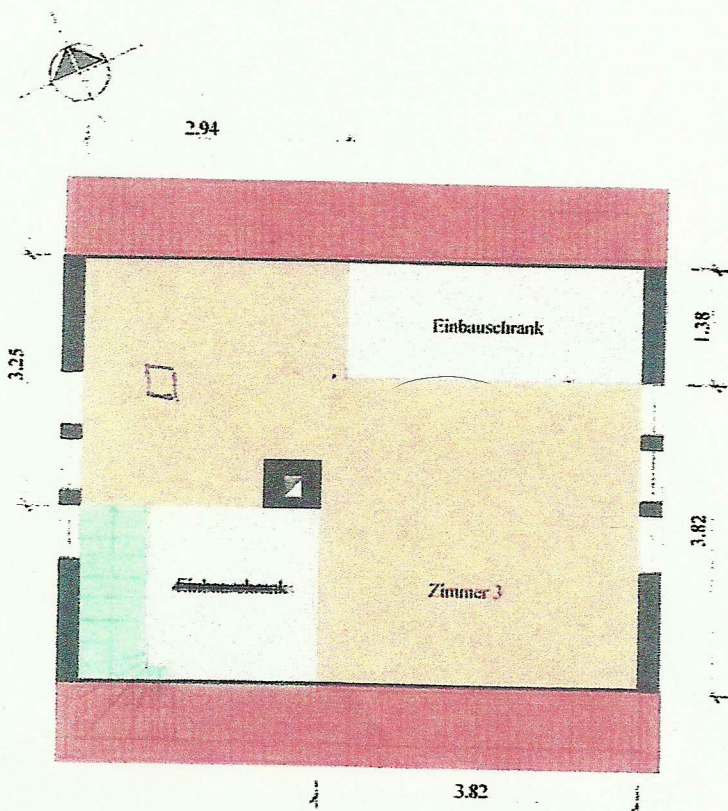
Wohnhaus/Grundriß DG
