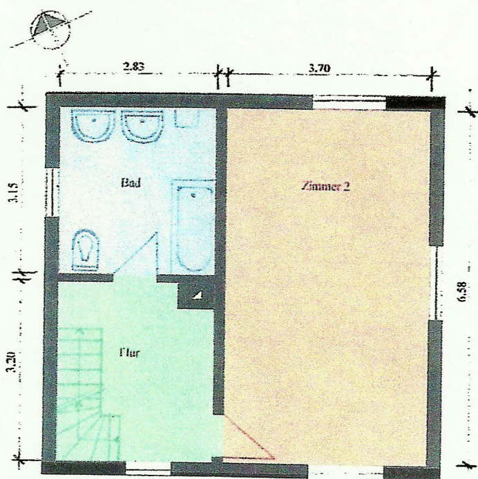
Wohnhaus/Grundriß OG
